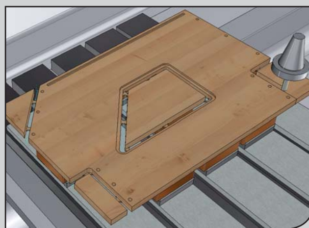
Optimisation du calibrage et des attaches.
